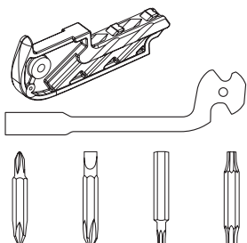
38. Bit-Schlüssel mit 39. – Innensechskant 5 mm für D-SUB Steckverbinder 40. – Innensechskant 4 mm für Bits 41. – Bit Torx 8 42. – Bit 6-kant 4 mm (Inbus) 43. Bit-Halter mit 44. – Bit Phillips 0 (Pozidrive) 45. – Bit Phillips 1 (Pozidrive) 46. – Bit Phillips 2 47. – Bit Schlitz 4 mm 48. – Bit Torx 10 49. – Bit Torx 15
